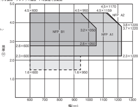
A101 床用鋼板・たてじま鋼板・プレメッキ鋼板 P12製造寸法範囲
