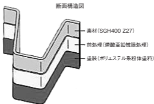
■塗装構造図
