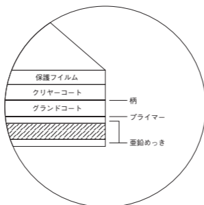
構成図 (一例)
