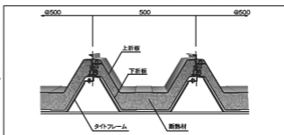
※下折板と上折板の裏面方向が逆になりますので、ご注意ください。
